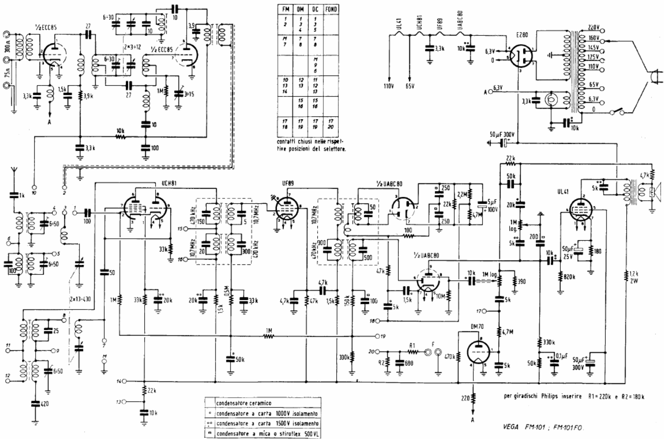
SCHEMA ELETTRICO DEL RADIORICEVITORE AM-FM VEGA MOD. FM-101 e FM-101FO
